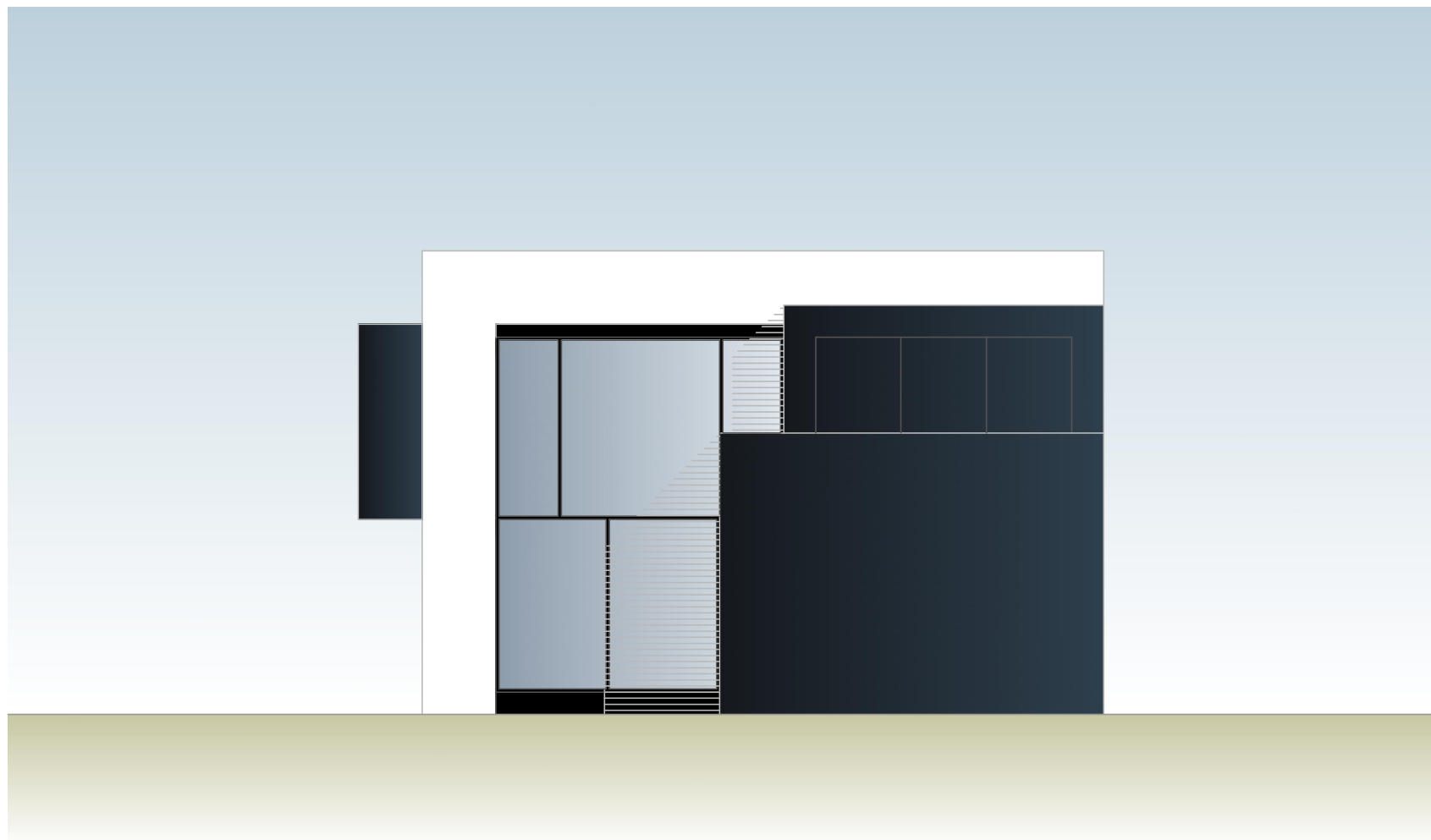
ALZADO SURESTE
